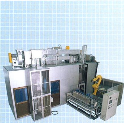
たて型蛍光管塗装乾燥装置
