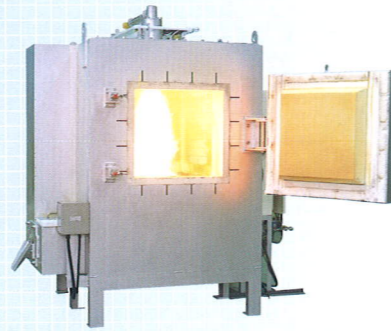
直燃式鉛再生炉
