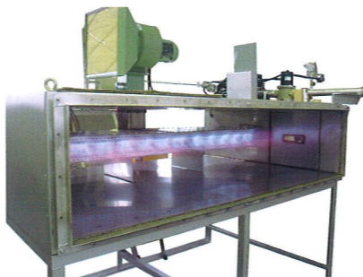
熱風発生器
